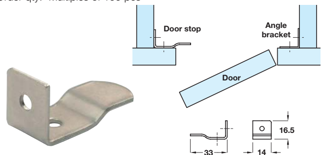
H Metal door stop
